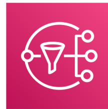
SNS
