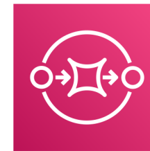
SQS
